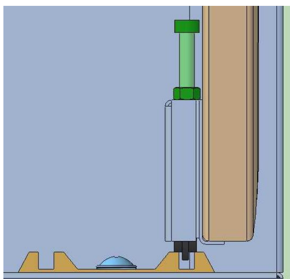
Рис. 1. Установка дверок.
