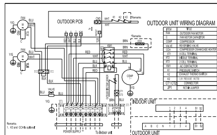
Схема для для наружных блоков (модель LCAC-48TI)
