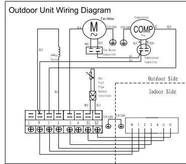
Схема для для наружных блоков (модель LCAC-18TI)
