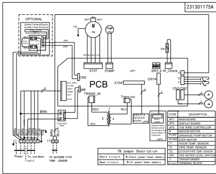
Схема для для внутренних блоков (модель LCAC-24TCI)
