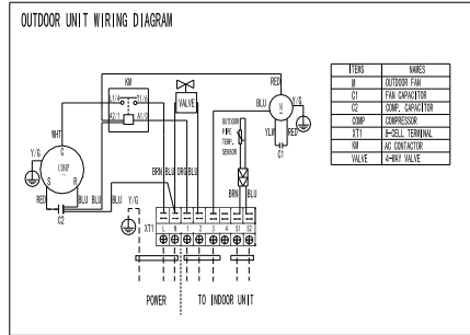
Схема для для наружных блоков (модель LCAC-24TI)
