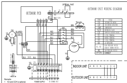
Схема для для наружных блоков (модель LCAC-36TI)
