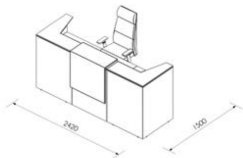
СТОЙКА РЕСЕПШЕН 2420x1500x1125
