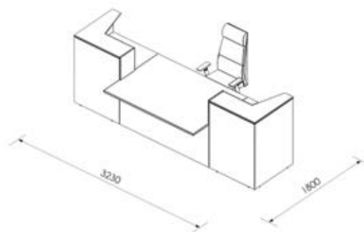
СТОЙКА РЕСЕПШЕН 3230x1800x1125
