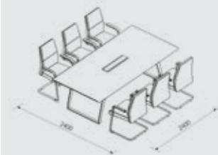
СТОЛ ДЛЯ ПЕРЕГОВОРОВ на 4 человека
