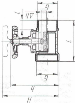
Рисунок 1 – Внешний вид клапанов угловых моделей КПКМ, КПК, КПК и КПКМ, КПКМ, КПКМ
