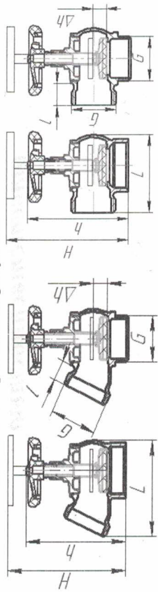
Исполнение 1: КПКМ, КПК, КПКМ. Исполнение 2: КПКМ, КПКМ, КПКМ
