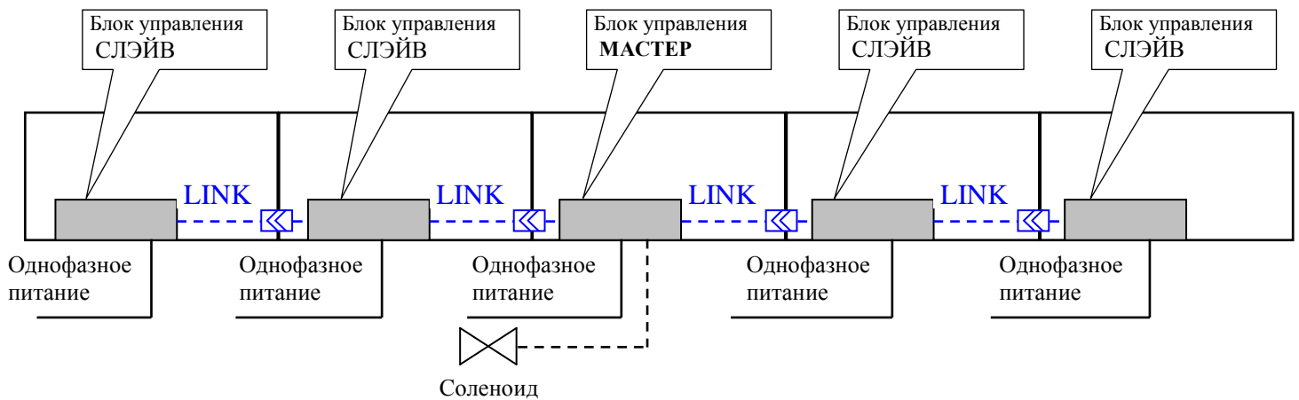
Рис. ПЗ. Схемы подключений оборудования при соединении витрин в линию.
