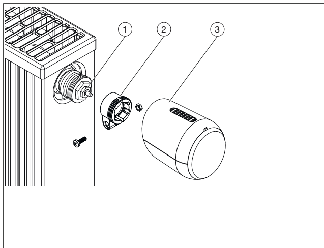
Рис. 4: монтаж „mote 200“
