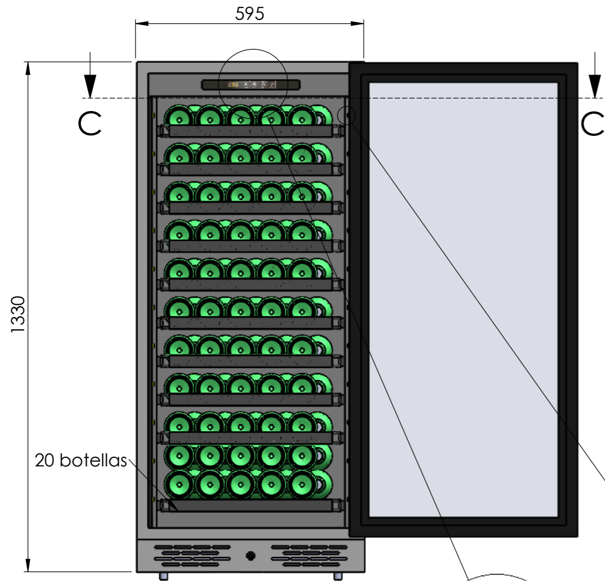
ALZADO
