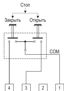
Схема для низковольтного управления электроприводом
