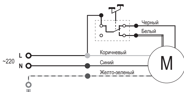
Схема подключения электропривода
