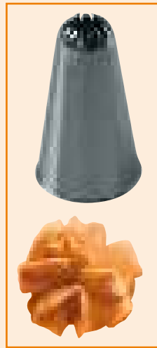
cod. size # BS 0195 Ø25 h40 Ø12 BS 0195K Ø25 h40 Ø14
